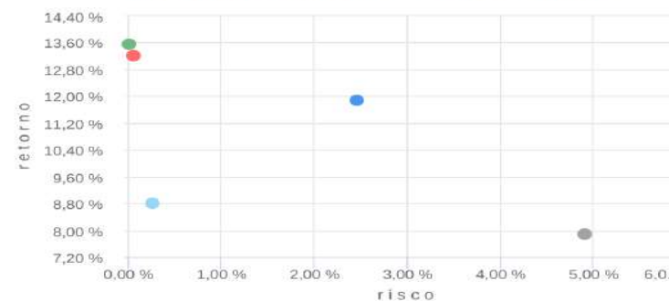
Risco x Retorno - 01/09/2022 a 31/08/2023 (diária)
